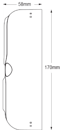
Vue Latérale
