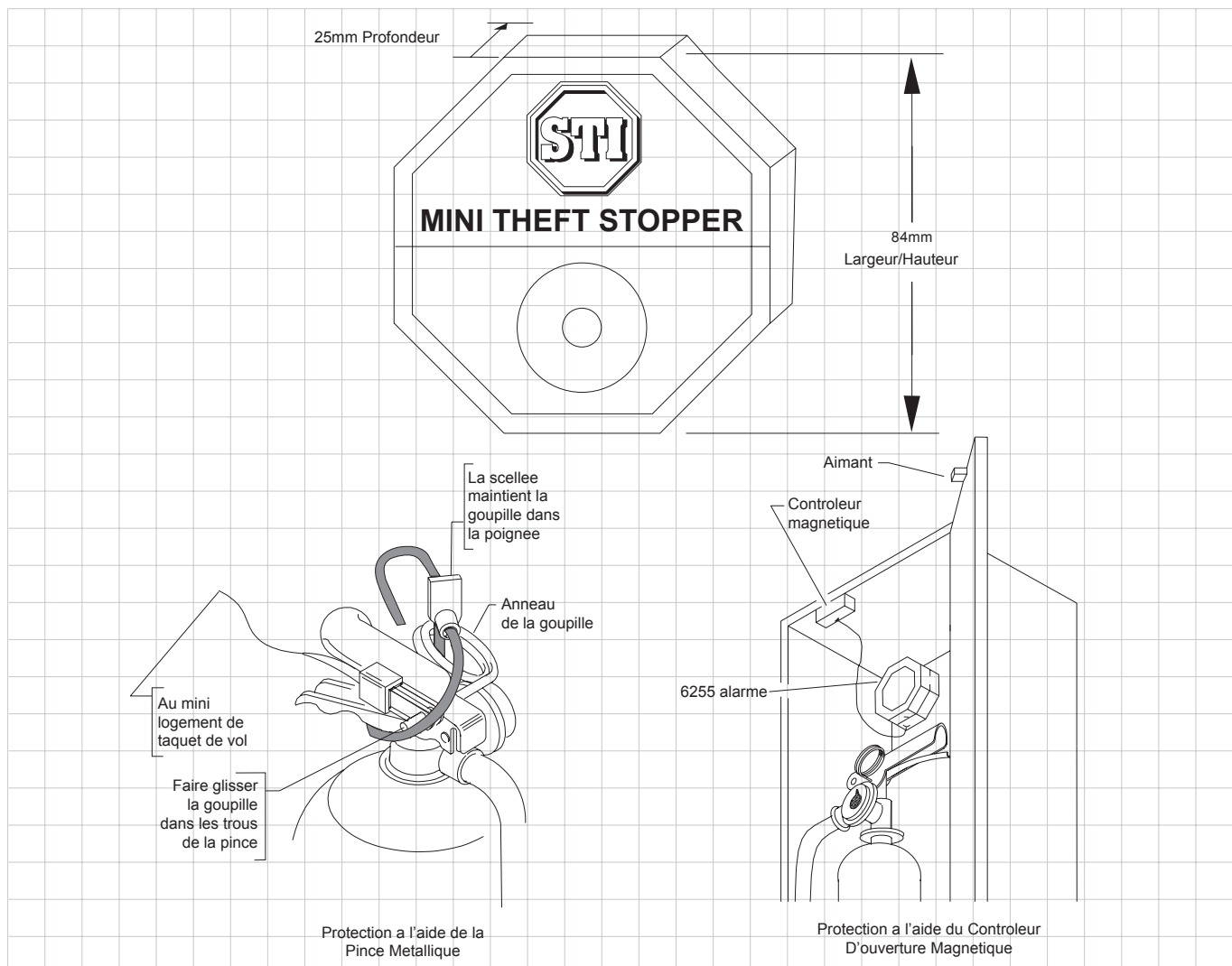
Pince en acier (KIT-131)
